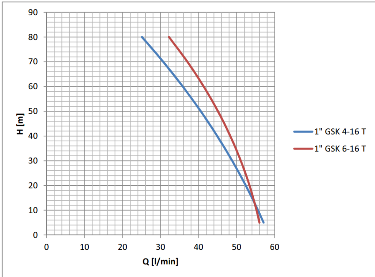
Grafická závislosť zodpovedá krivke 1" GSK 4-16 T
